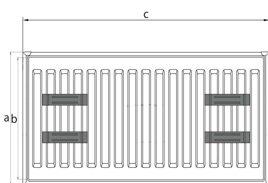
4 кронштейна | 4 hangers; 400/...../1600 mm
