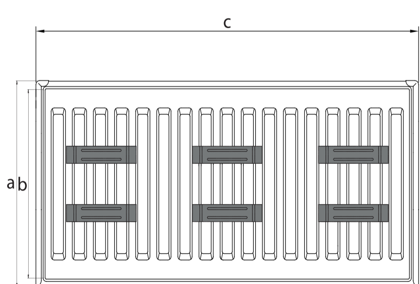
6 кронштейнов | 6 hangers; 1700/...../2000 mm
