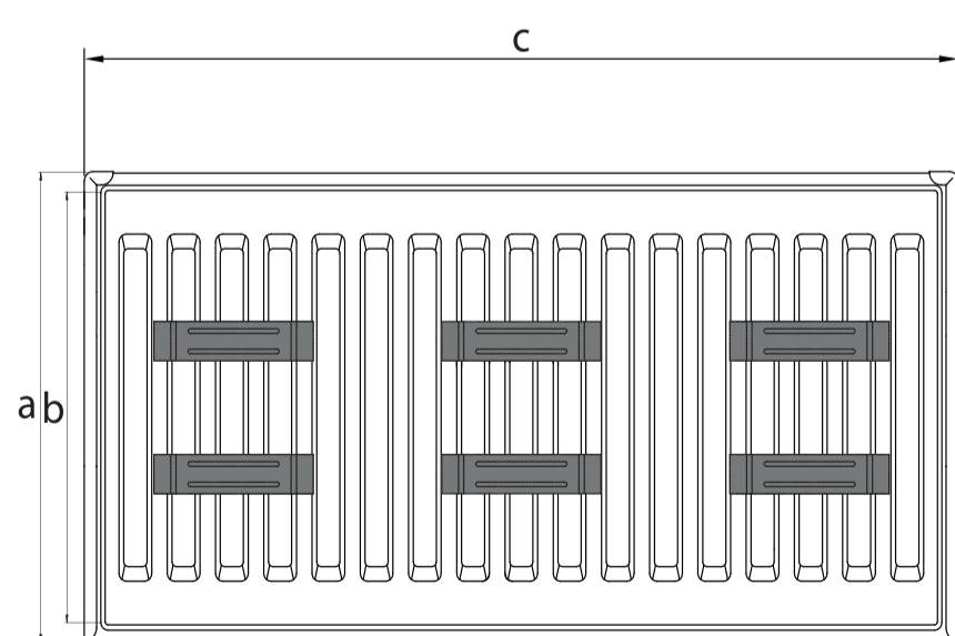
6 кронштейнов | 6 hangers; 1700/...../3000 mm
