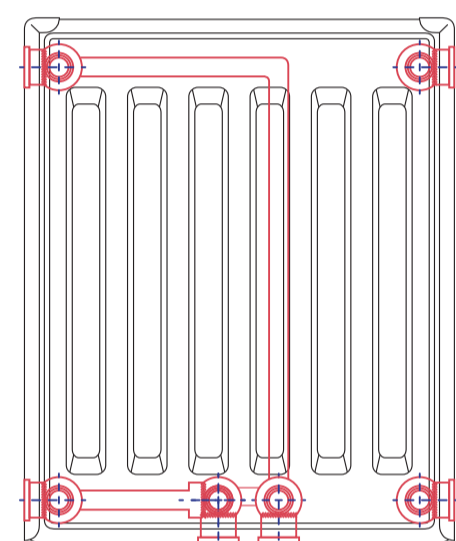
Компактное соединение на 6 отверстий с С-образным кронштейном 6 Holes Compact Middle Connection
