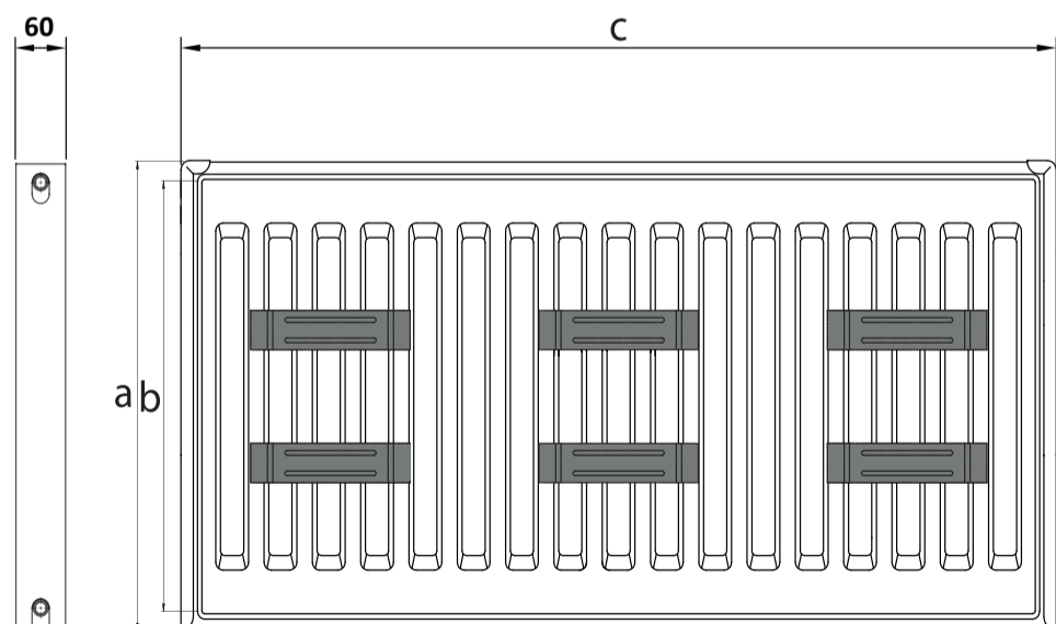
6 кронштейнов | 6 hangers; 1700/...../2000 mm
