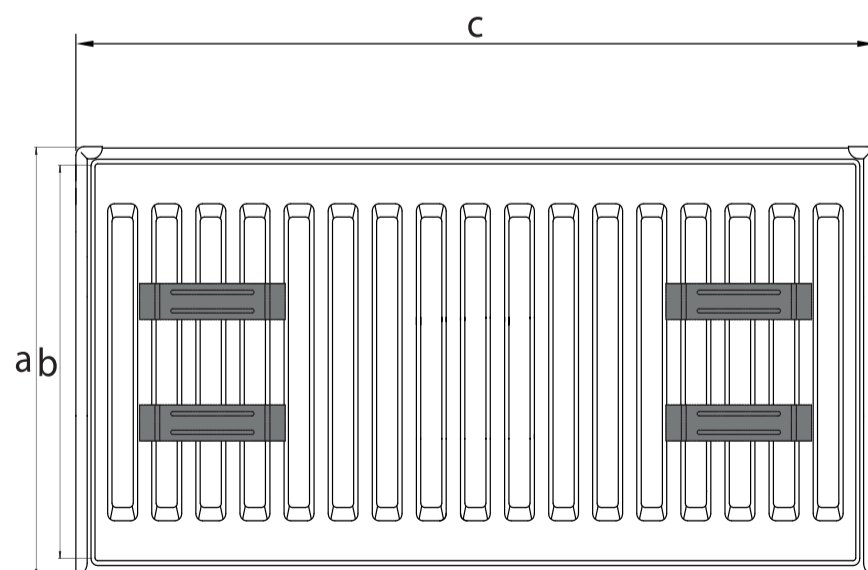
4 кронштейна | 4 hangers; 400/...../1600 mm
