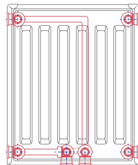
Компактное соединение на 6 отверстий с С-образным кронштейном
