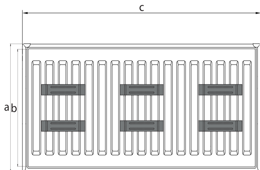
6 кронштейнов | 6 hangers; 1700/...../3000 mm
